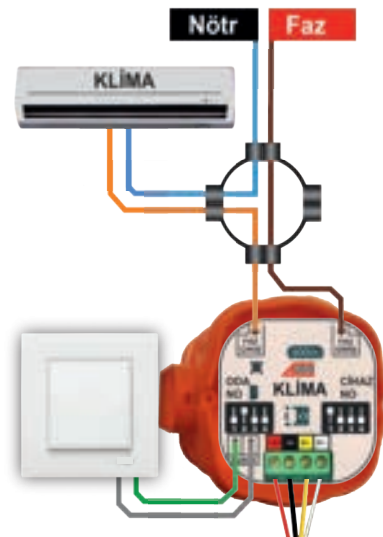
OTOMASYON KABLOSU(OK-4)
