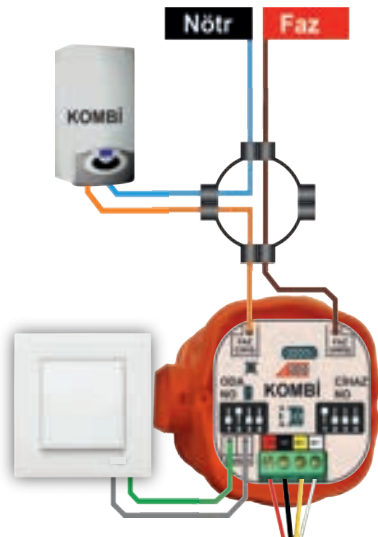
KOMBİ BAĞLANTISI
